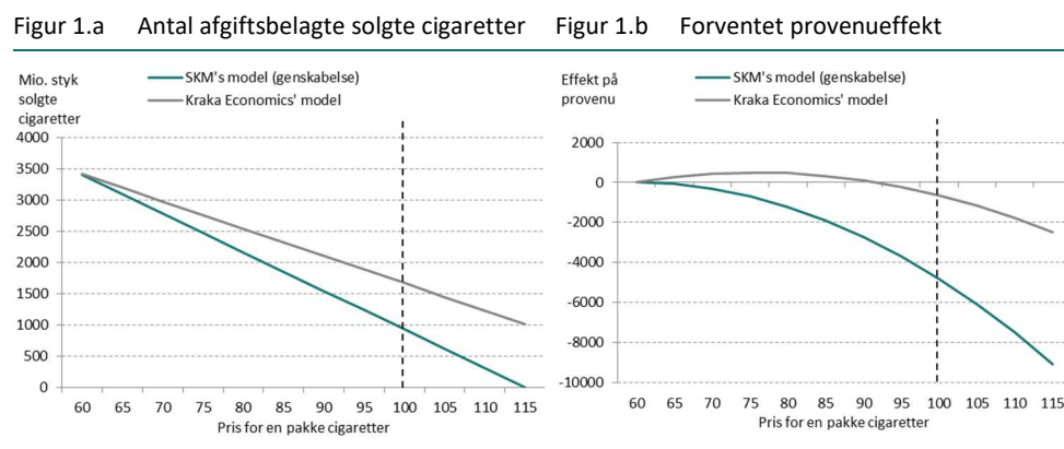
Figur 1 Forventet antal solgte afgiftsbelagte indenlandske cigaretter og forventet provenueeffekt ved forskellige cigaretpakkepriser
